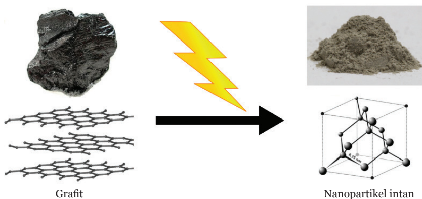
Gambar 8.7 Nanopartikel Intan
