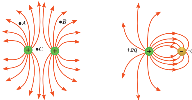
Gambar 4.6 Garis Gaya Listrik Dua Muatan
