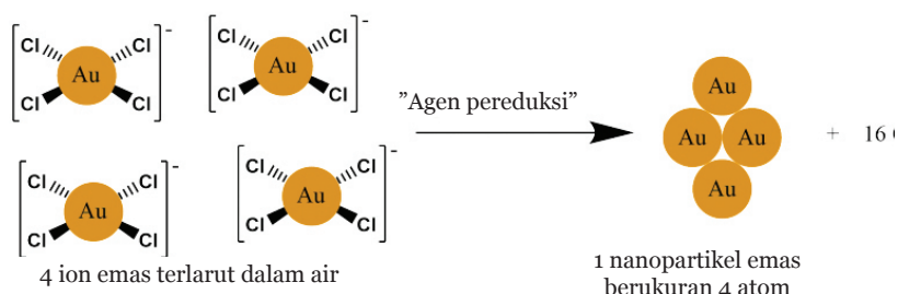
Gambar 8.6 Nanopartikel Emas
