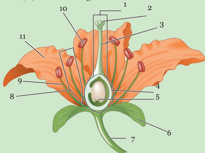
Gambar 2.1 Struktur Bunga
