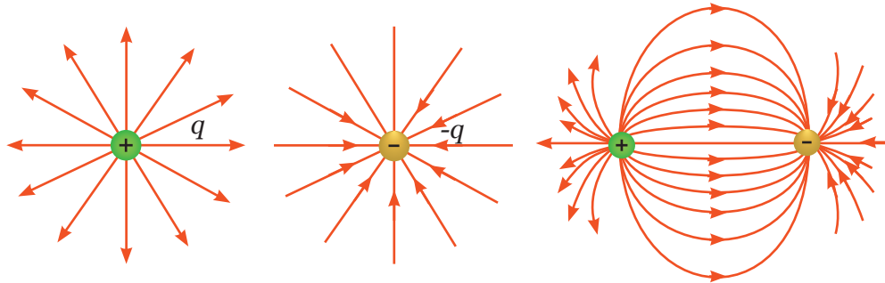
Gambar 4.5 Garis Gaya Listrik Dua Muatan
