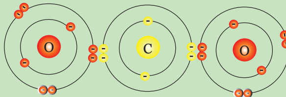
Gambar 8.5 Penggunaan Pasangan Elektron Bersama pada CO_2
