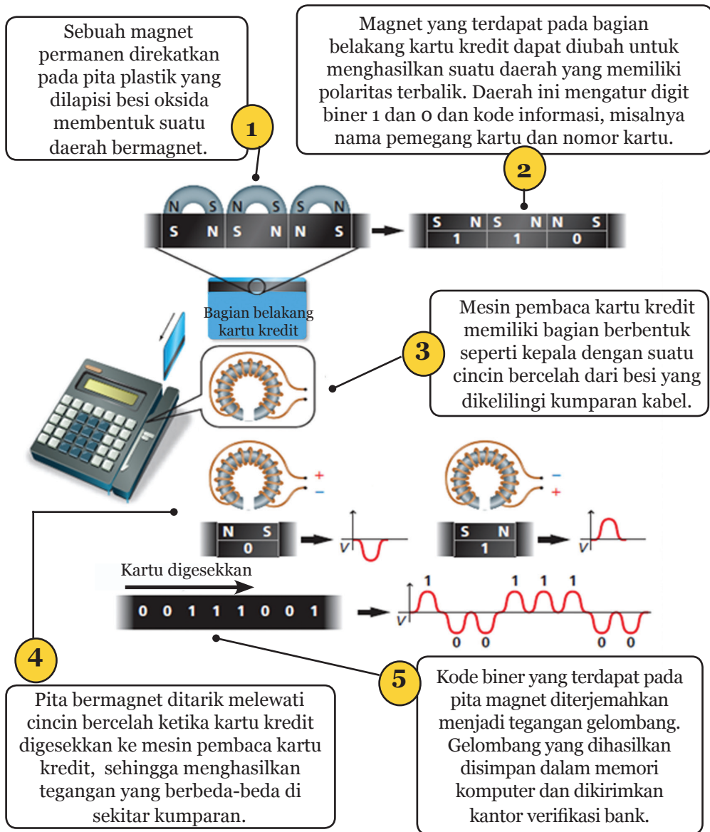
Gambar 6.1 Cara Kerja Kartu Kredit dan Mesin Pembaca Kartu Kredit
