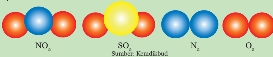
Gambar 8.1 Model Atom Dalton Beberapa Molekul
