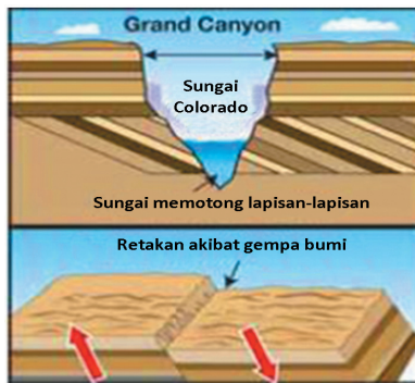
Gambar 9.3 Ilustrasi Terjadinya Lapisan Tanah secara Lateral
