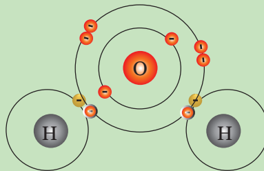
Gambar 8.4 Penggunaan Pasangan Elektron Bersama pada H_2O
