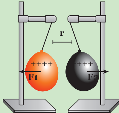
Gambar 4.3 Ilustrasi Gaya Tolak Menolak Dua Balon yang Bermuatan
