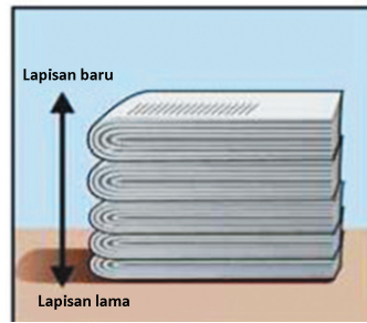
Gambar 9.1 Ilustrasi Terjadinya Superposisi. Tampak seperti Tumpukan Koran, Semakin ke Atas Merupakan Lapisan Baru
