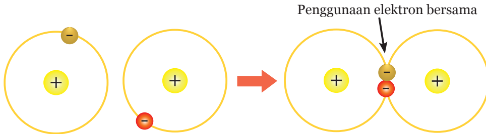
Gambar 8.3 Penggunaan Elektron Bersama pada Molekul H_2
