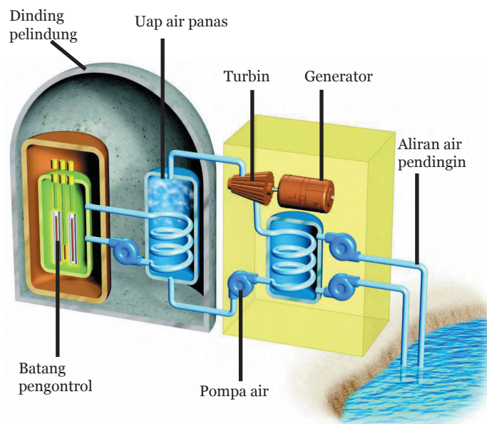
Gamba 10.1 Skema Teknologi pada Pembangkit Listrik Tenaga Nuklir
